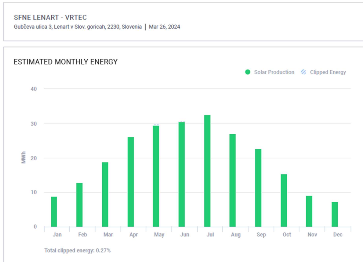
Slika 6-6: Mesečna simulacija delovanja
