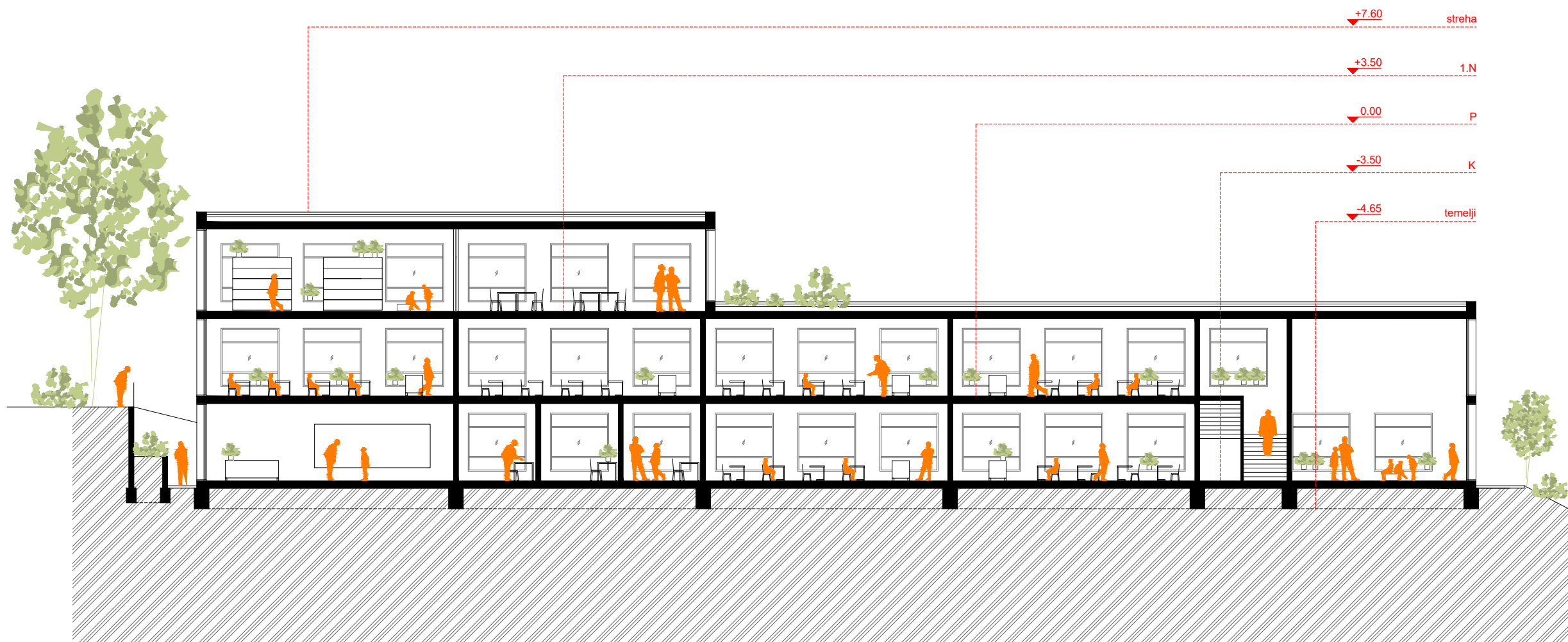
VZDOLŽNI PREREZ B-B 2.8
